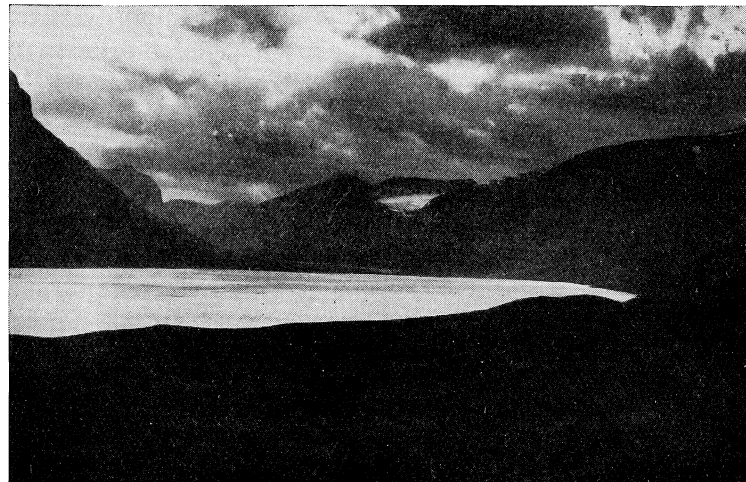
FRÅN BACKARNA ÖSTER OM SARVESJOKKS MYNNING ALKAJAURE OCH ALKAVAGGE.
