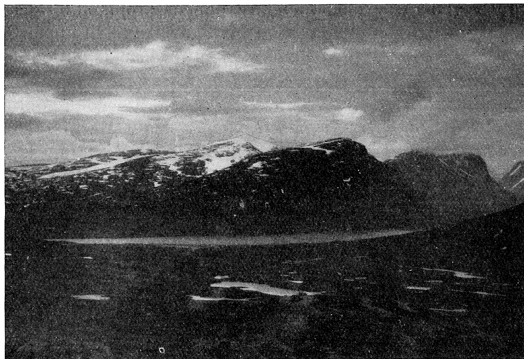
UTSIKT FRÅN UNNA RISSAVARE MOT ALKAJAURE OCH ALKAVARE.
